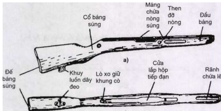
Hình 13: Súng
