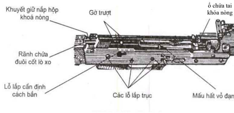
Hình 21: Hộp khoá nòng
