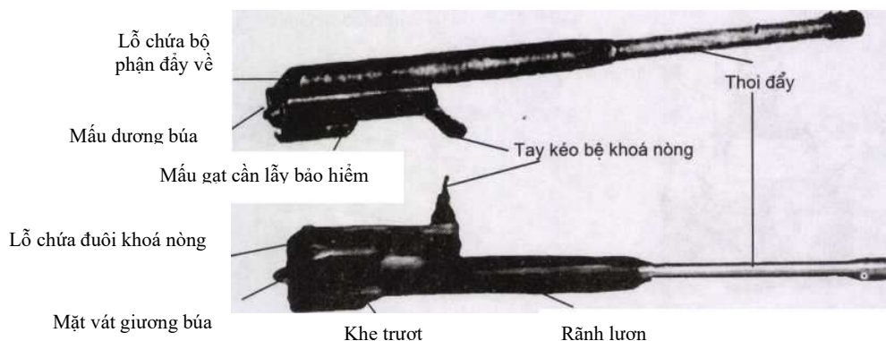
Hình 23: Bộ khoá nòng
