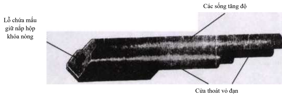
Hình 22: Nắp hộp khoá nòng
