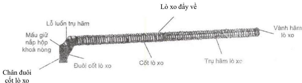
Hình 26: Bộ phận đẩy về
