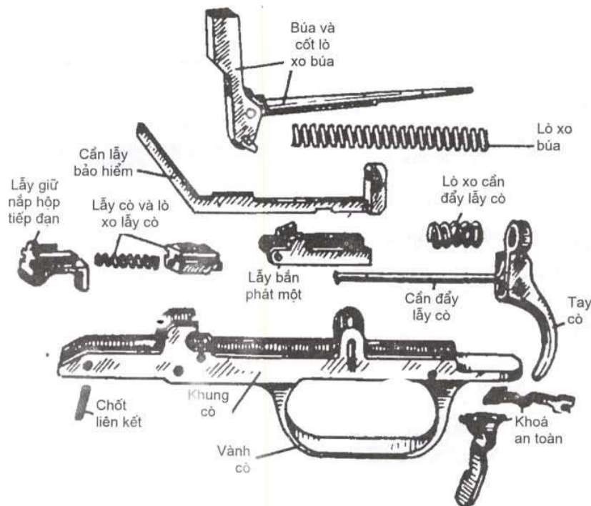
Hình 9: Bộ phận cò
