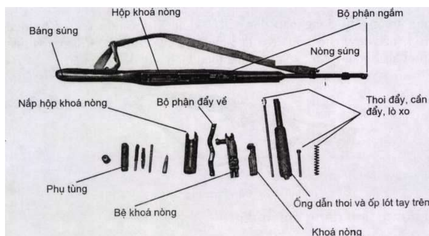
Hình 2: Cấu tạo của súng trường CKC
