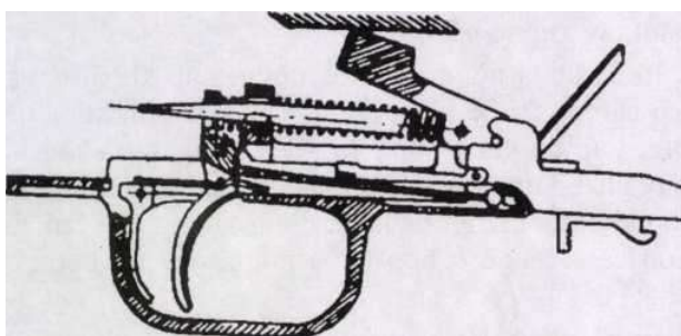
Hình 17: Chuyển động các bộ phận khi bắn
