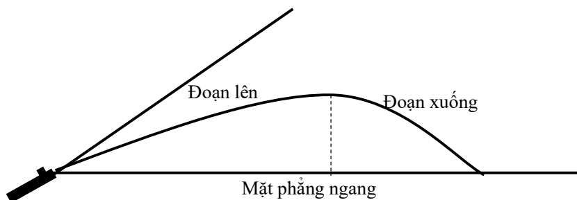
Hình 48: Đường đạn trong không gian
