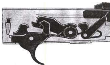
Hình 33: Vị trí các chi tiết bộ phận cò khi bắn phát một
