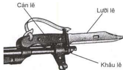
Hình 30: Lưỡi lê
