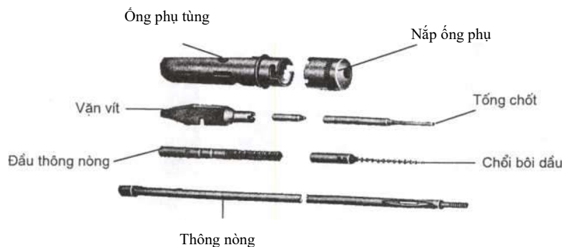
Hình 31: Phụ tùng
