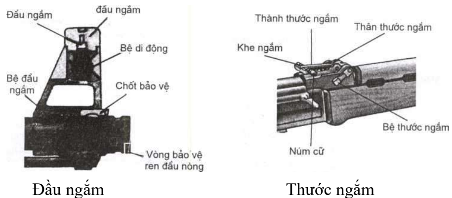
Hình 20: Bộ phận ngắm
