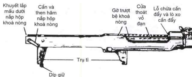
Hình 5: Hộp khoá nòng
