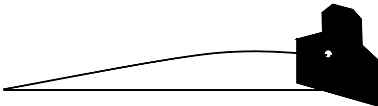
Hình 47: Quỹ đạo đường đạn
